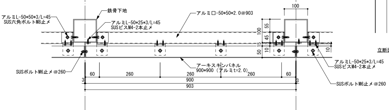
平断面詳細図 (鉄骨) S=1/10
