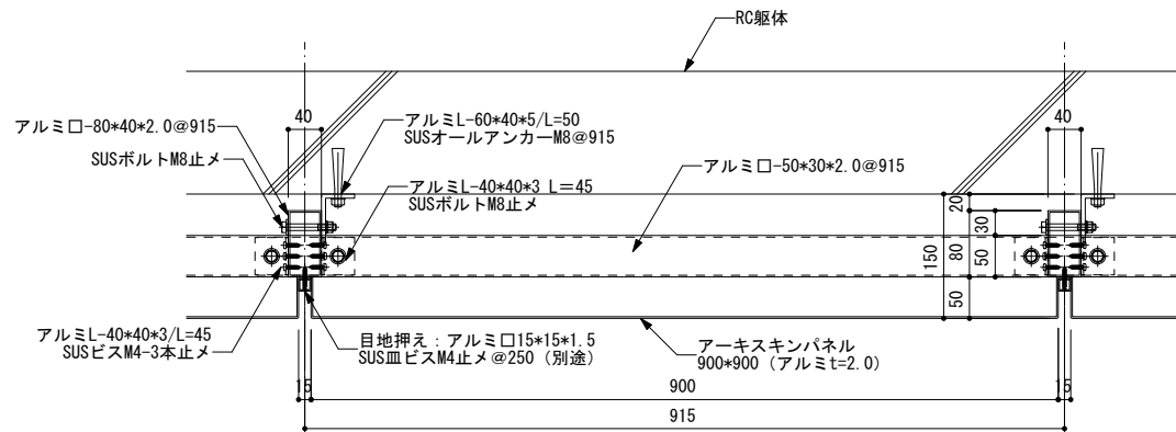
平断面詳細図 (RC) S=1/10
