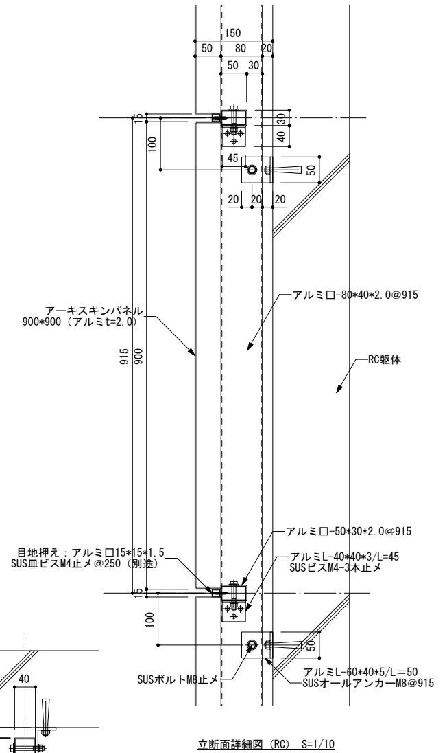
立断面詳細図 (RC) S=1/10
