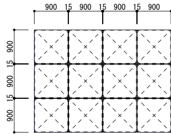
立面图 S=1/100
