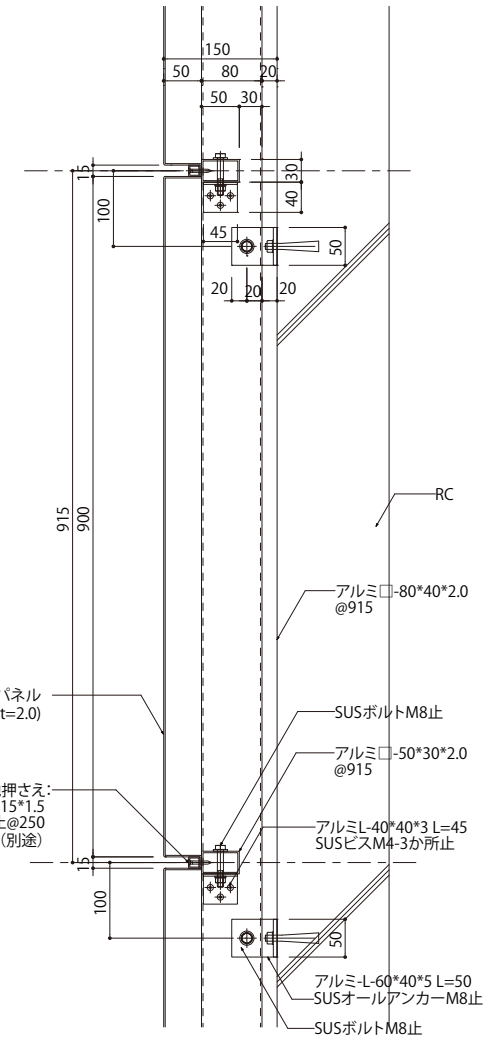
立断面詳細図 (RC) S=1/10
