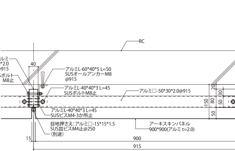
平断面詳細図 (RC) S=1/10
